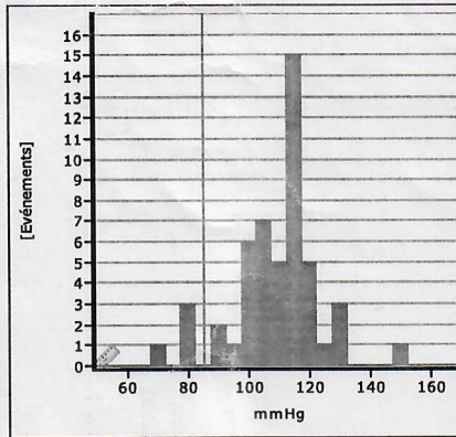
Diastolique Réveil
