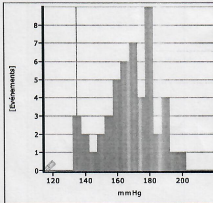
Systolique Réveil
