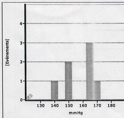
Systolique Endormi
