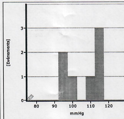
Diastolique Endormi
